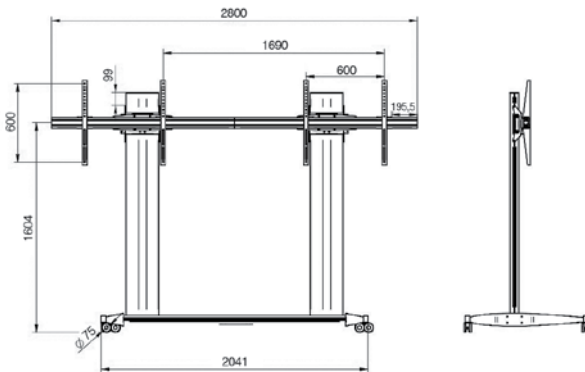
Optional support for screen tilting Montanti opzionali per il tilting degli schermi
